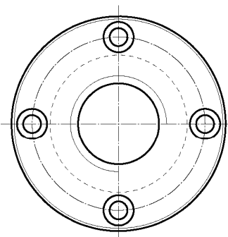
Fino a Tr 22x5 (4 fori)
