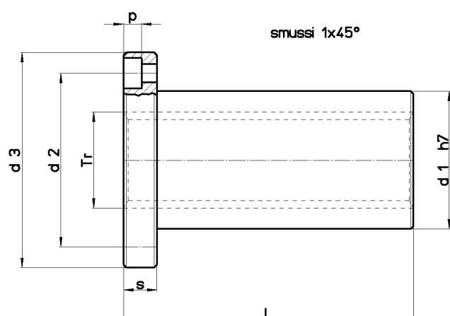
Da Tr 25x5 (6 fori)
