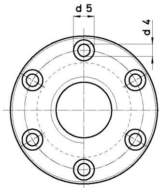
Da Tr 25x5 (6 fori)
